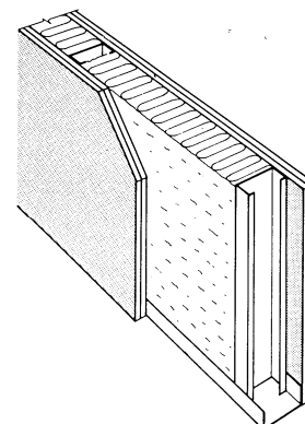
Fig. 1 Prinsipiell oppbygning av skillevegg med enkelt stenderverk.
